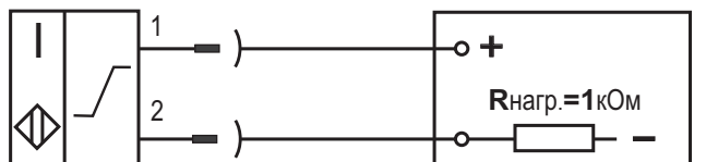
Схема подключения к оборудованию
